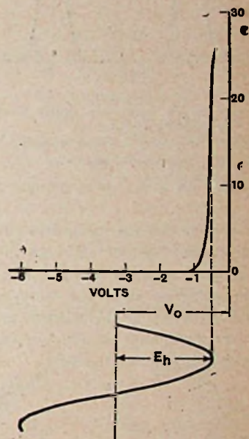
Fig. 2. Verticaal is de stroom i die door de diode gaat, in \mu A uitgezet, horizontaal de spanning op de diode in volts.
