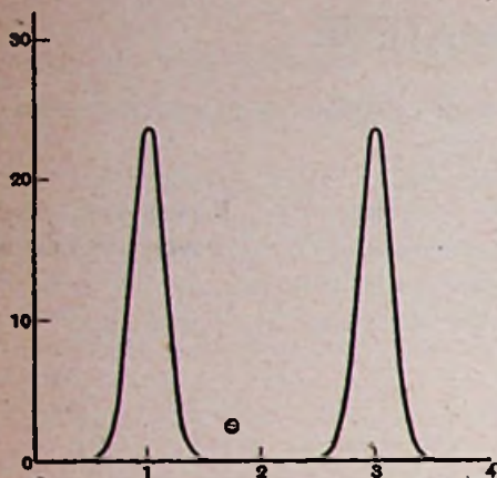
Fig. 3. De stroompieken, die in een normale diode optreden onder invloed van een wisselspanning.
