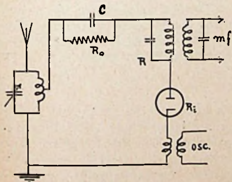
Fig. 1. Principeschema van een superingang met diode als menglamp.
